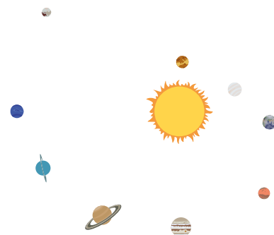
zonnestelsel
