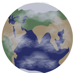
Aarde
