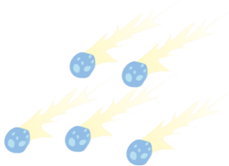
vallende sterren
