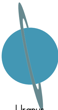
Uranus
