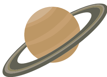
Saturnus
